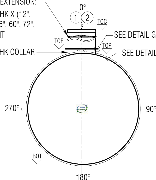
ELEVATION B
