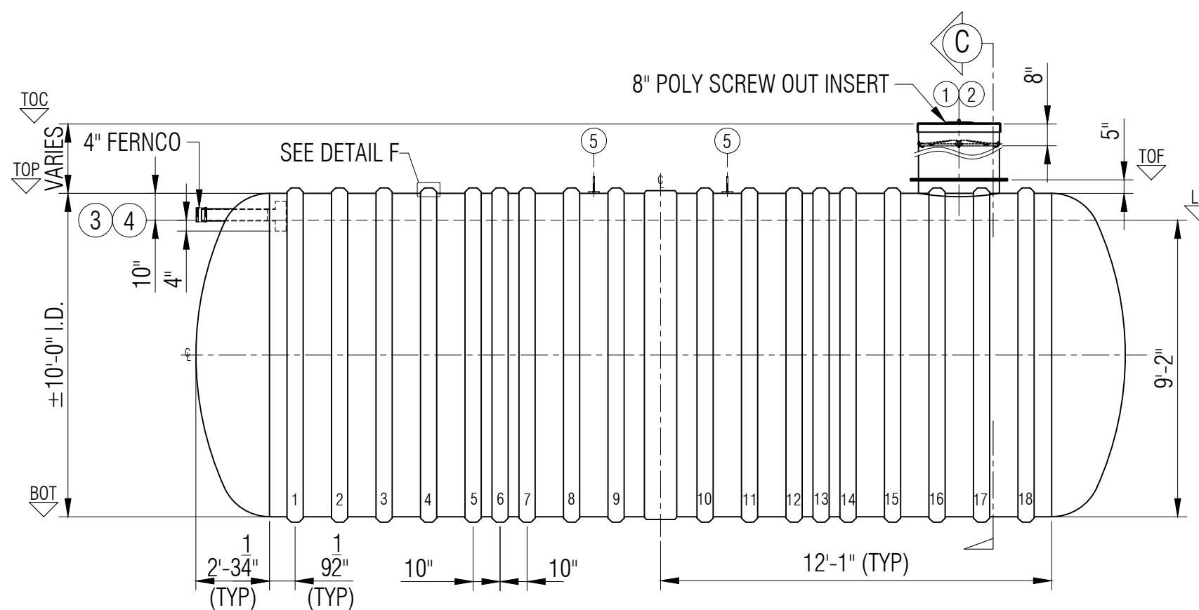
ELEVATION A
