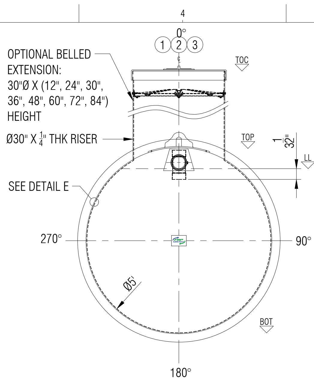
ELEVATION B
