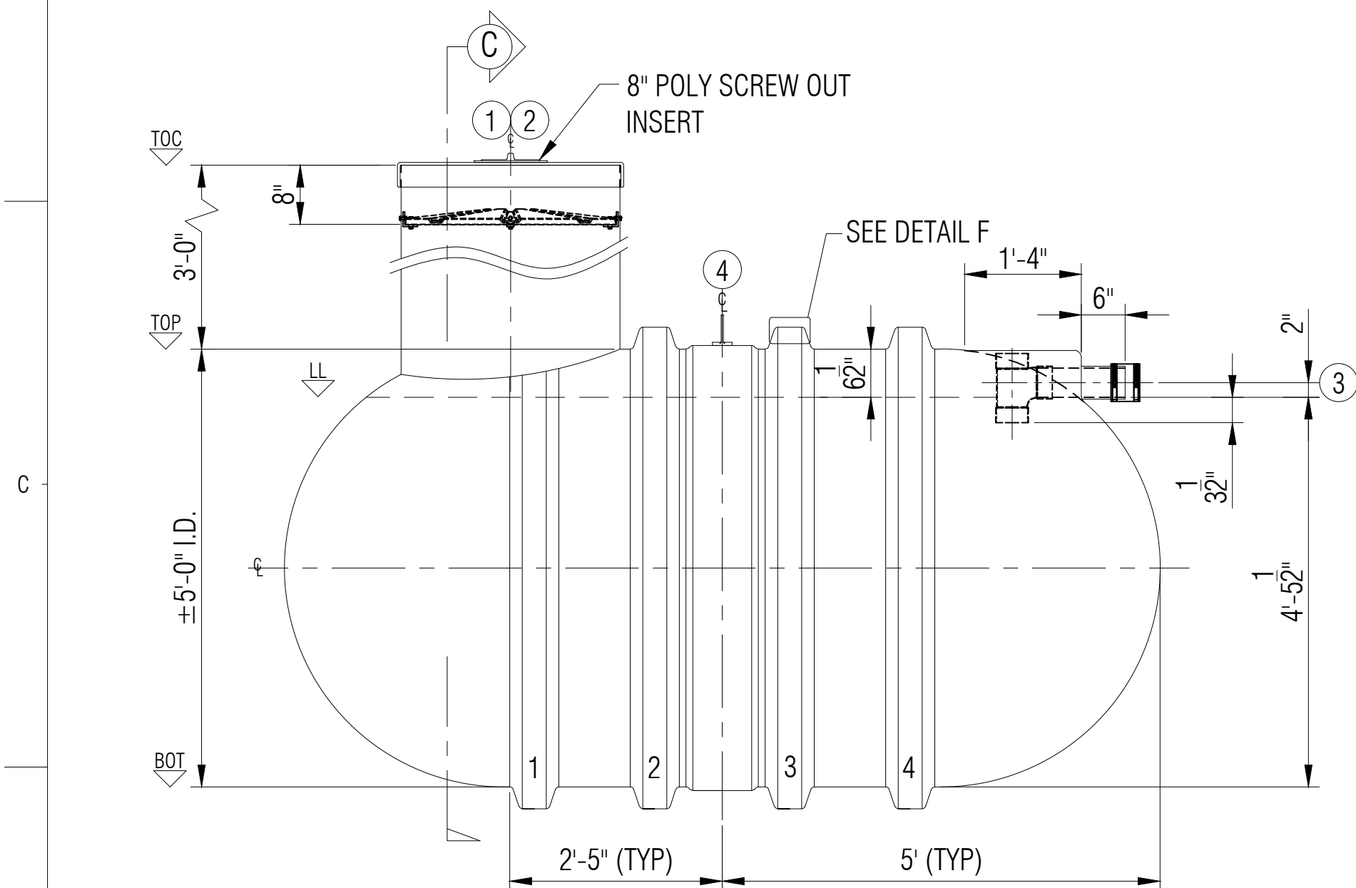
ELEVATION A
