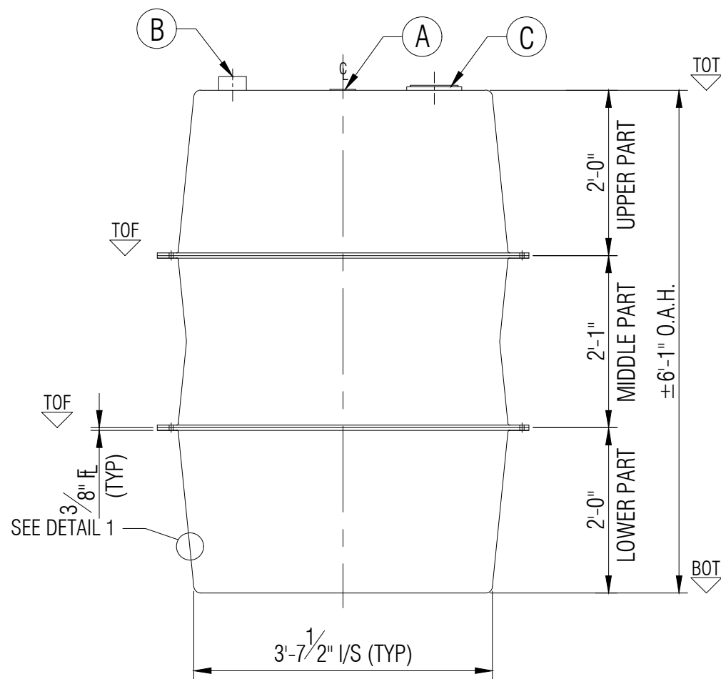
ELEVATION A
