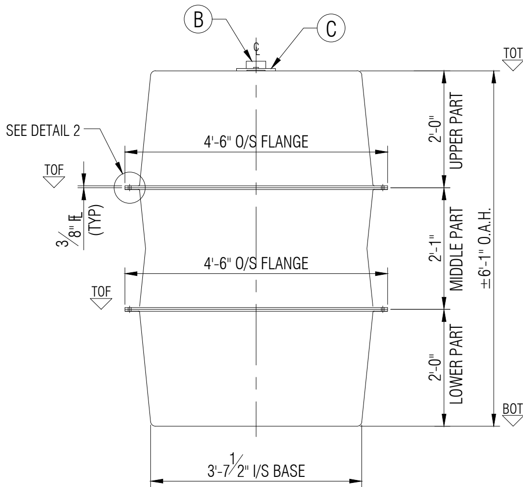
ELEVATION B
