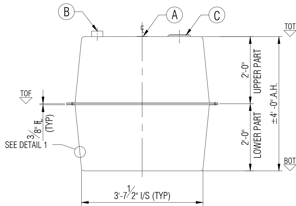
ELEVATION A
