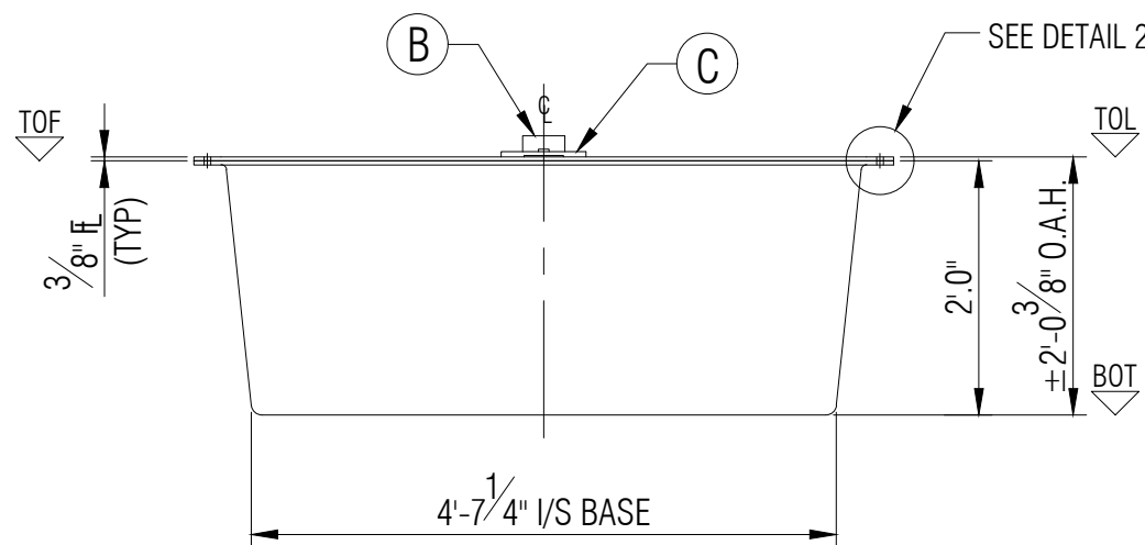
ELEVATION B
