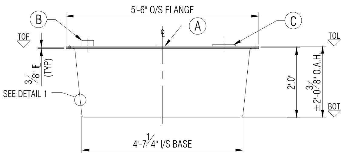
ELEVATION A
