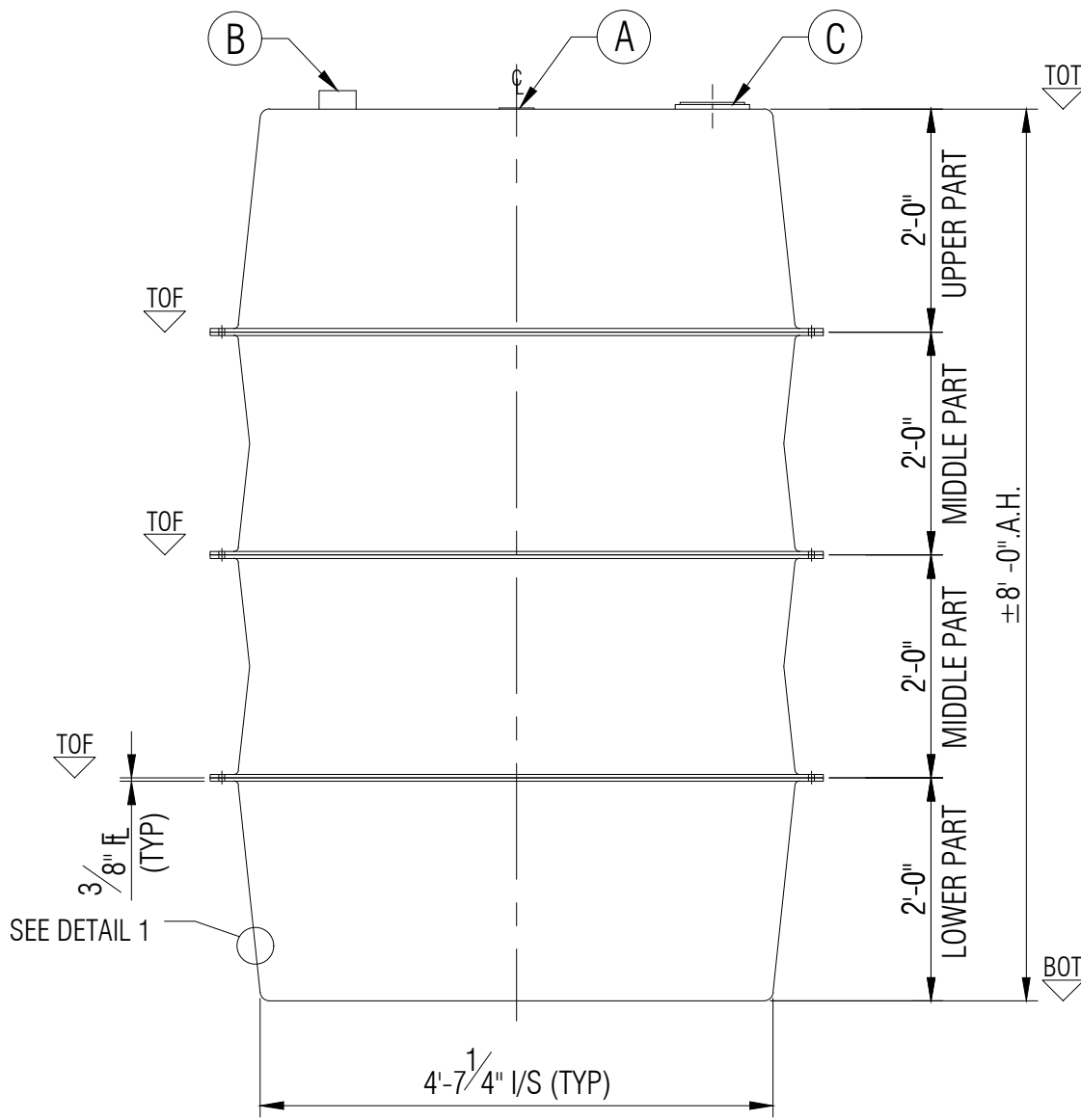
ELEVATION A
