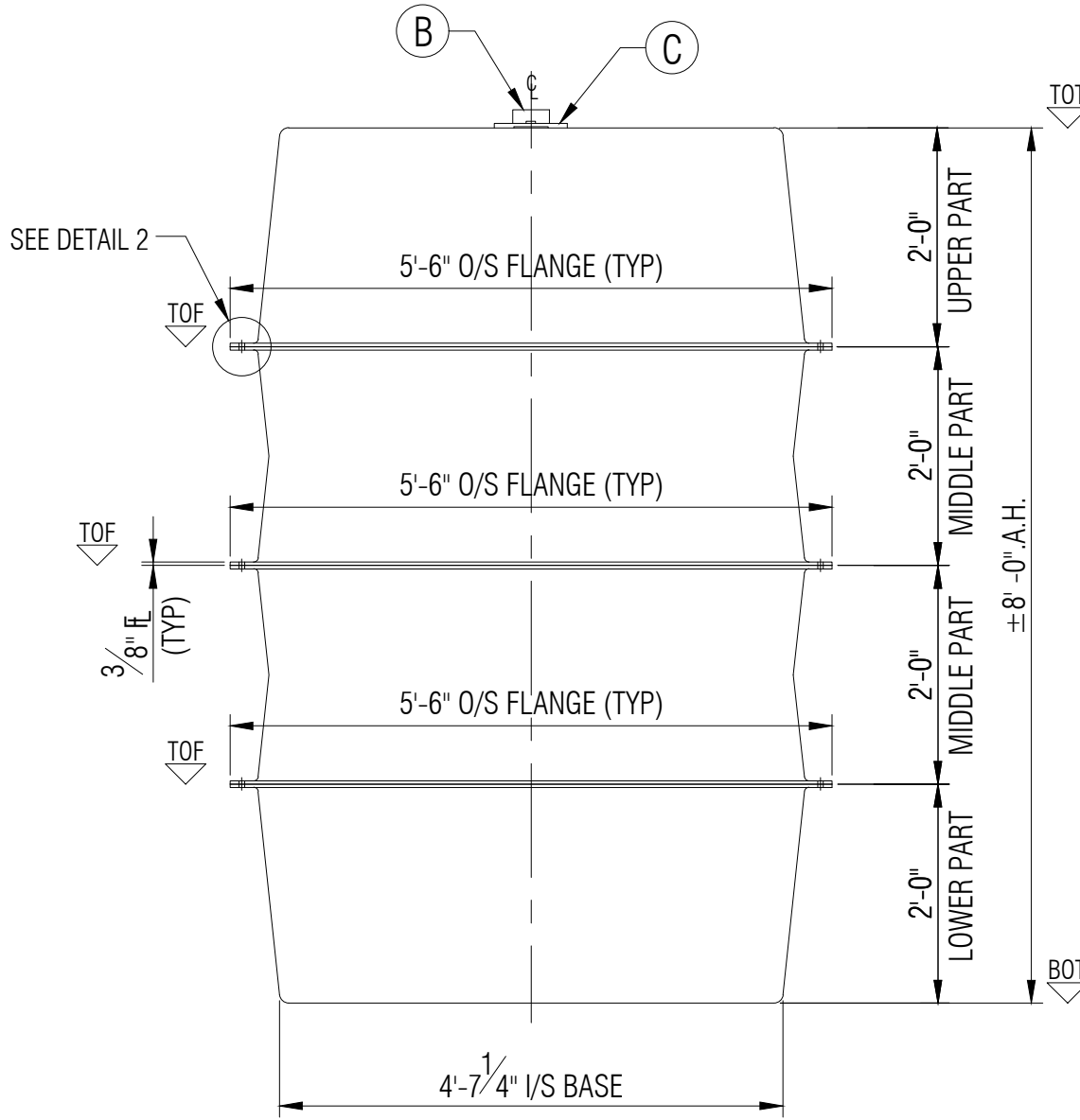
ELEVATION B
