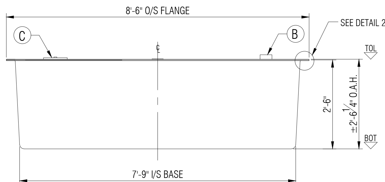
ELEVATION B
