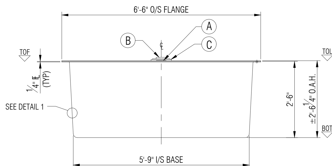
ELEVATION A
