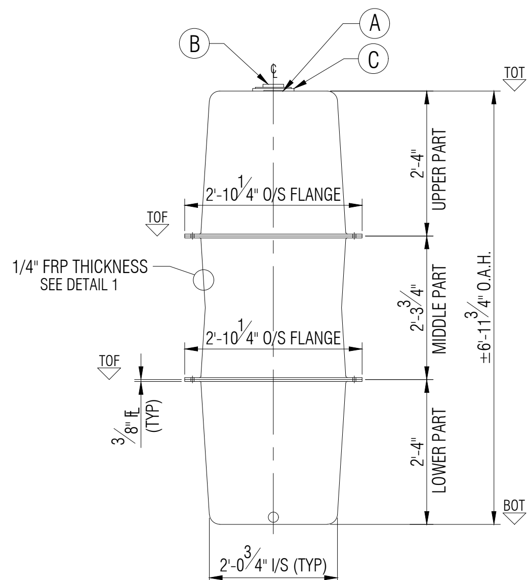
ELEVATION A
