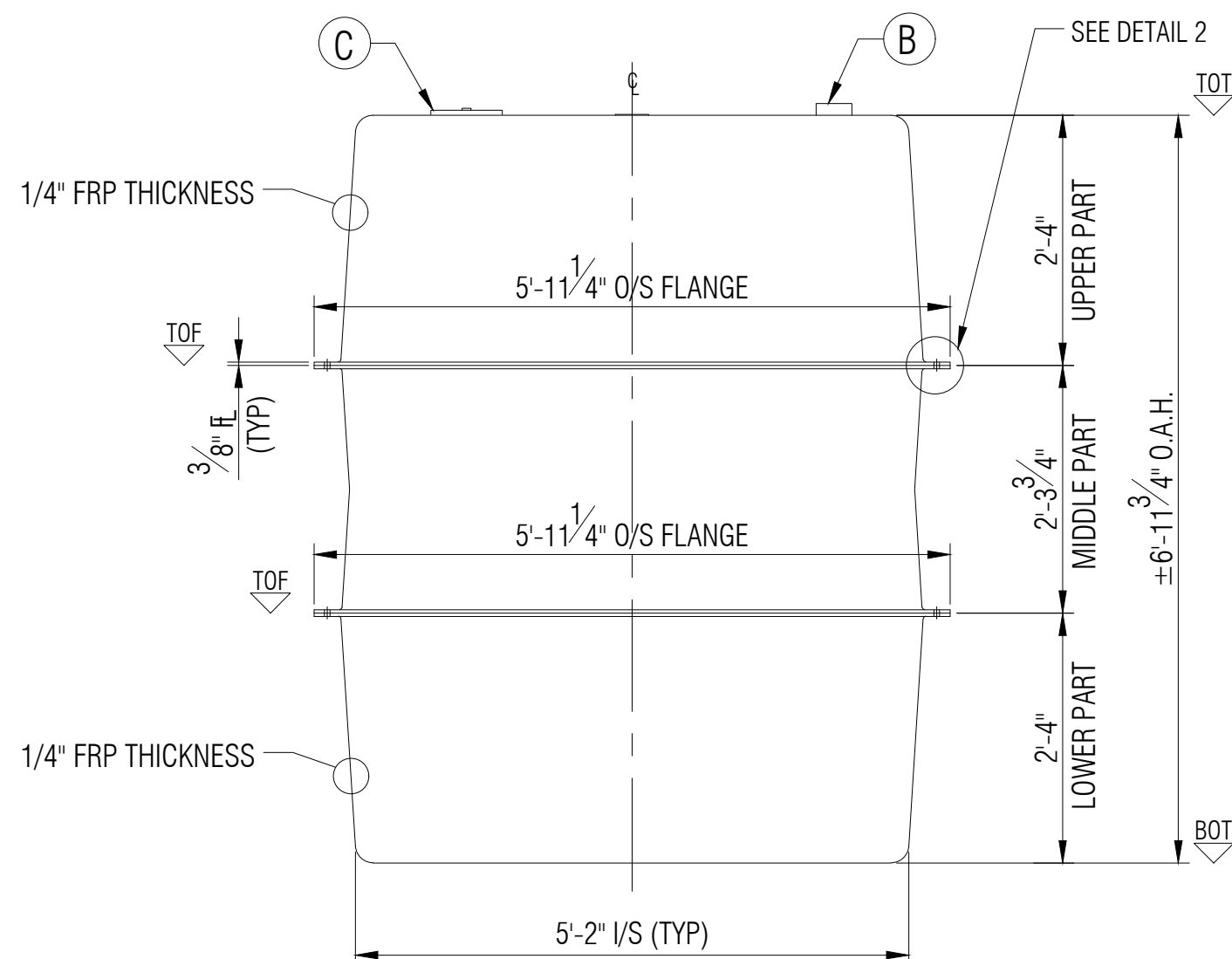
ELEVATION B
