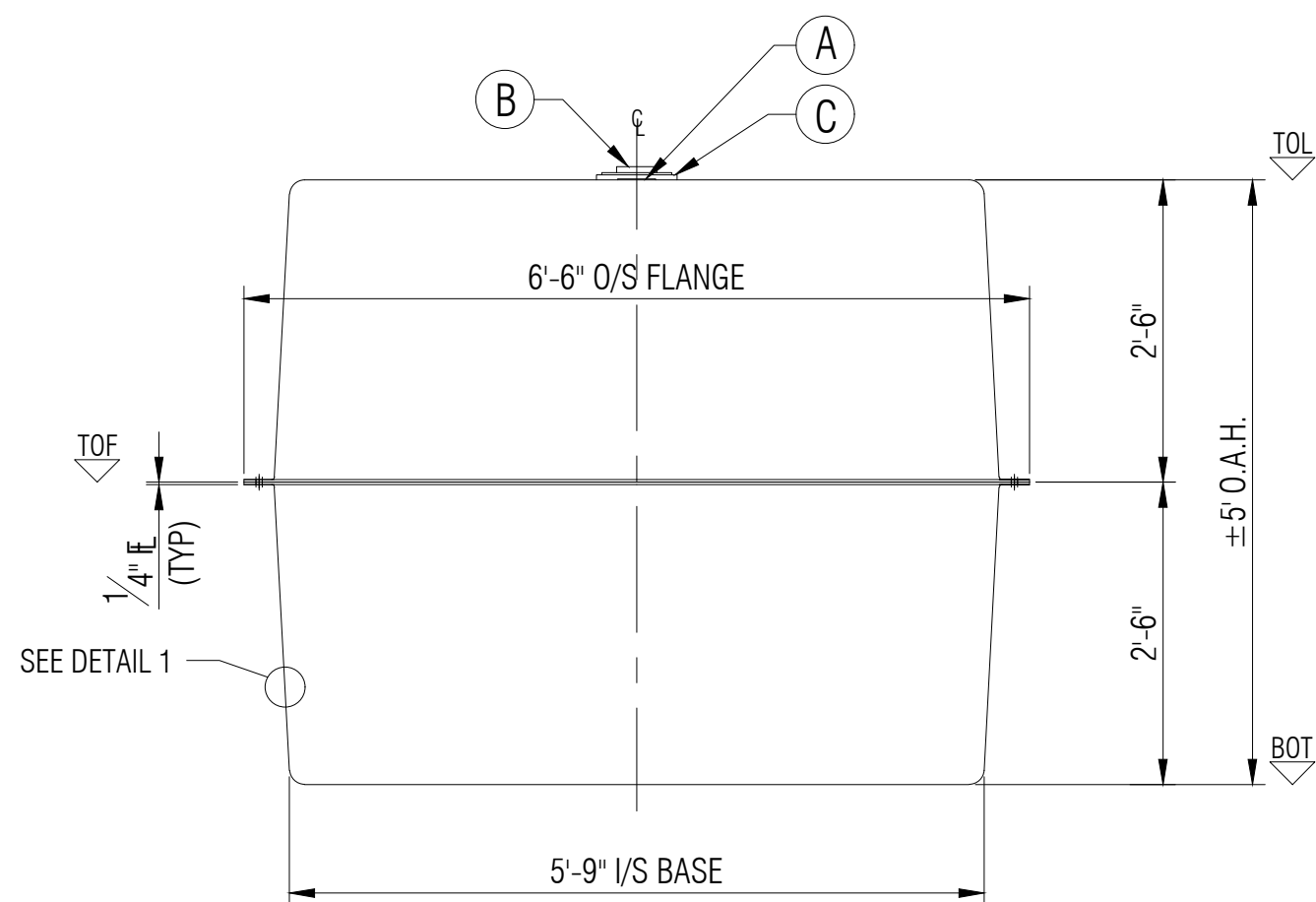
ELEVATION A
