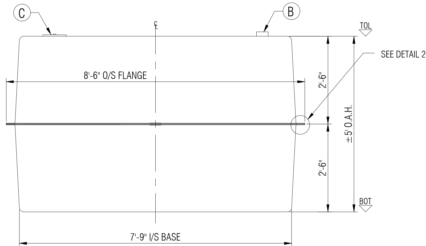
ELEVATION B
