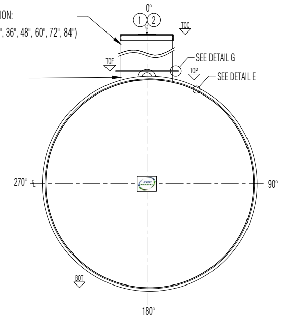
ELEVATION B
