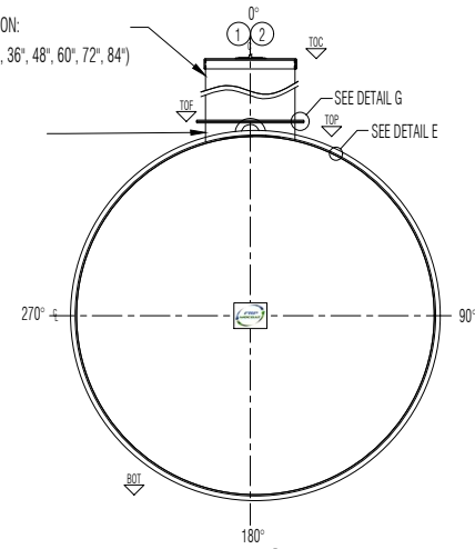
ELEVATION B
