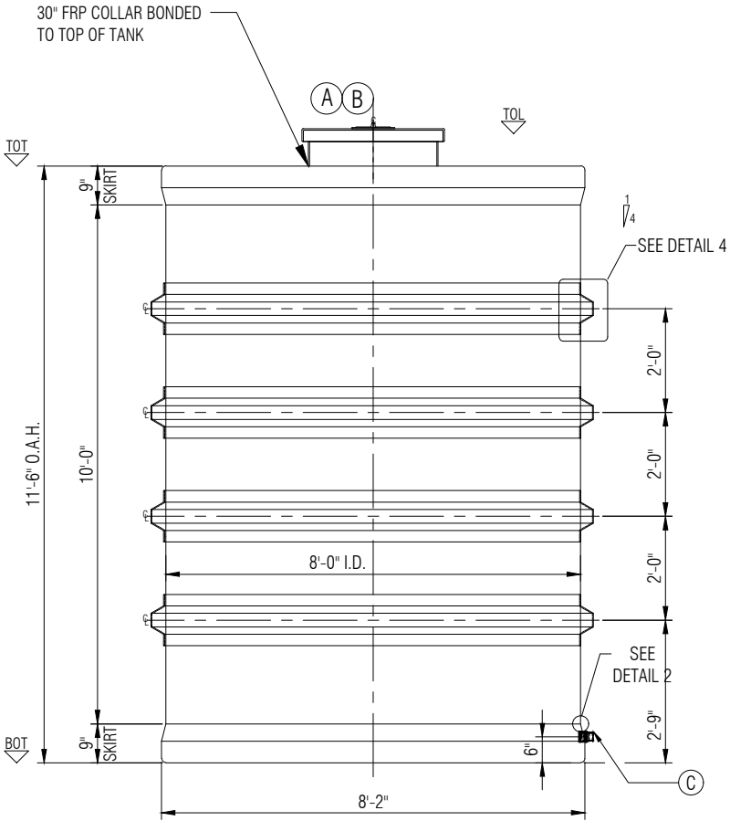
ELEVATION B
