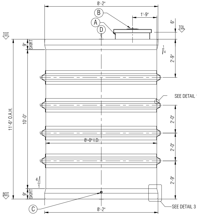
ELEVATION A
