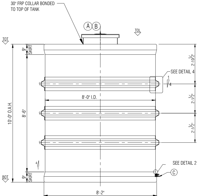
ELEVATION A
