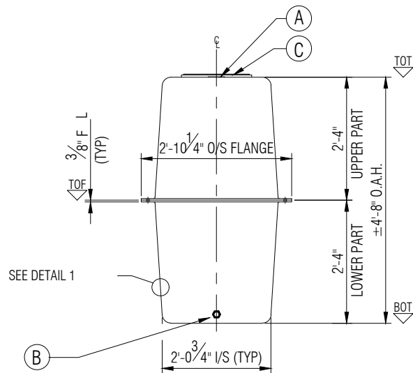
ELEVATION A
