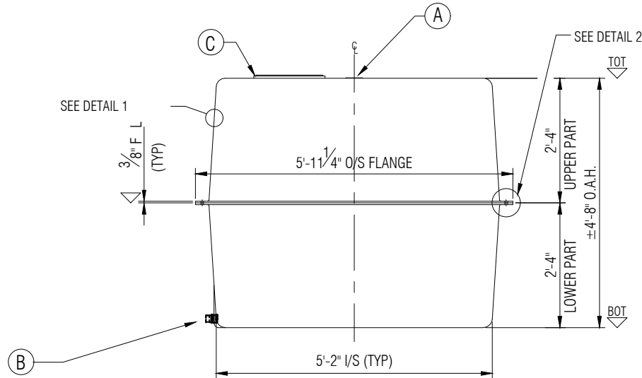
ELEVATION B
