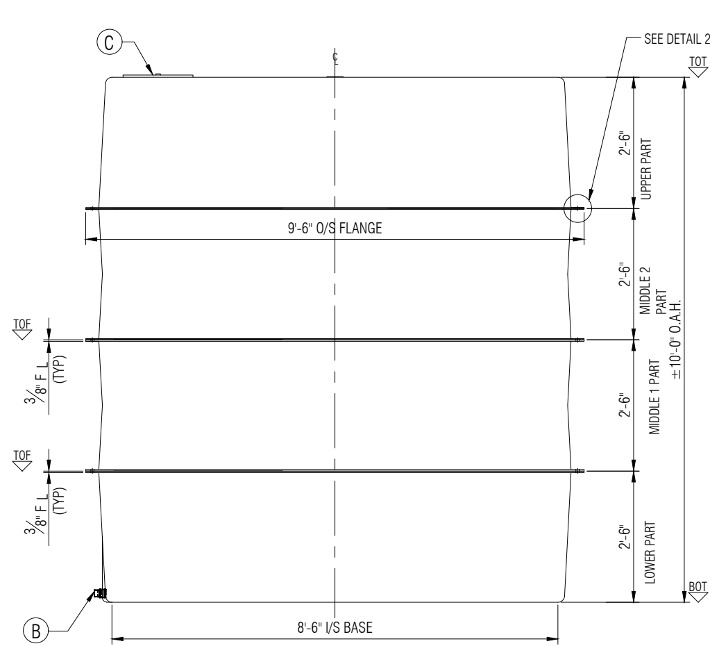
ELEVATION B
