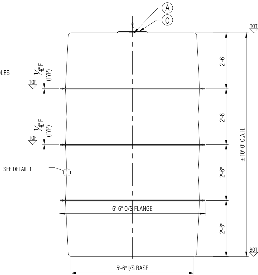
ELEVATION A
