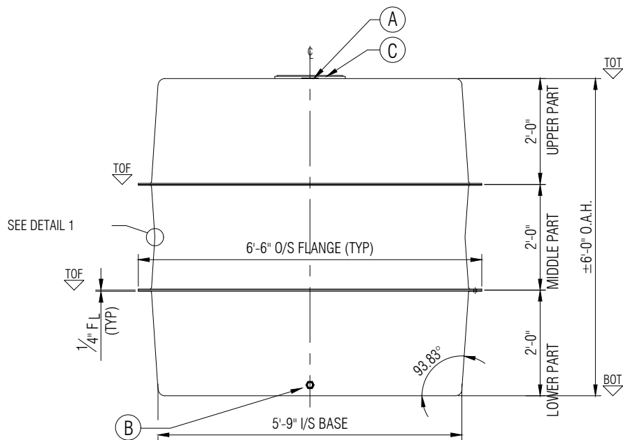
ELEVATION A
