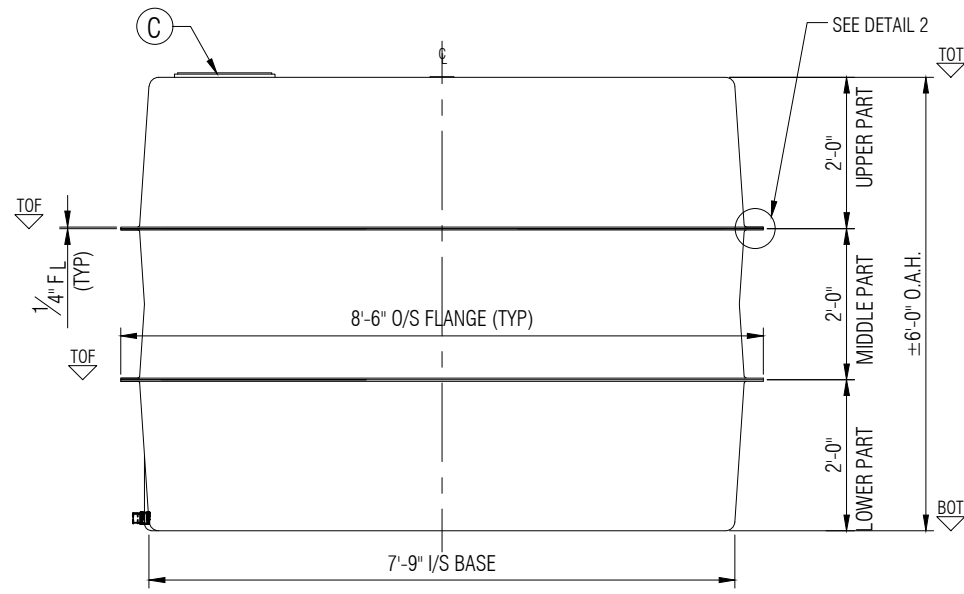
ELEVATION B
