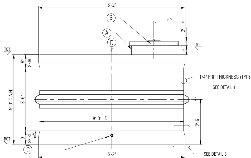
ELEVATION A
