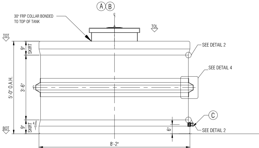
ELEVATION B
