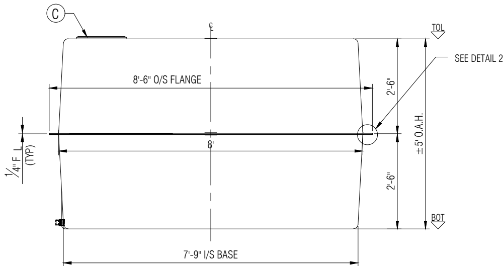
ELEVATION B
