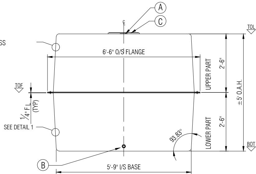
ELEVATION A
