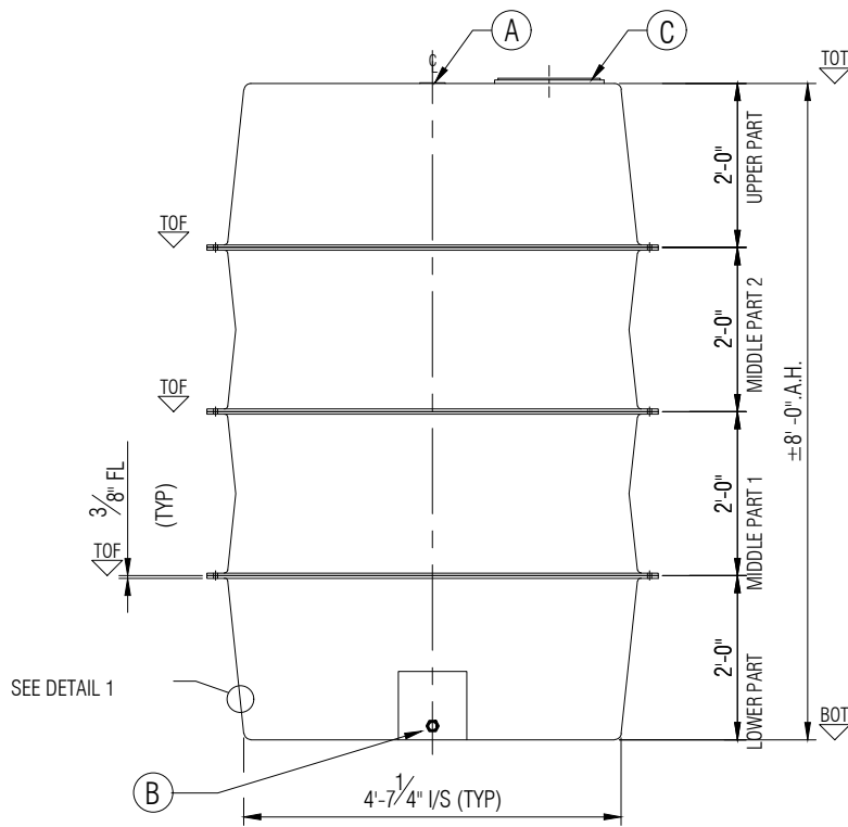
ELEVATION A
