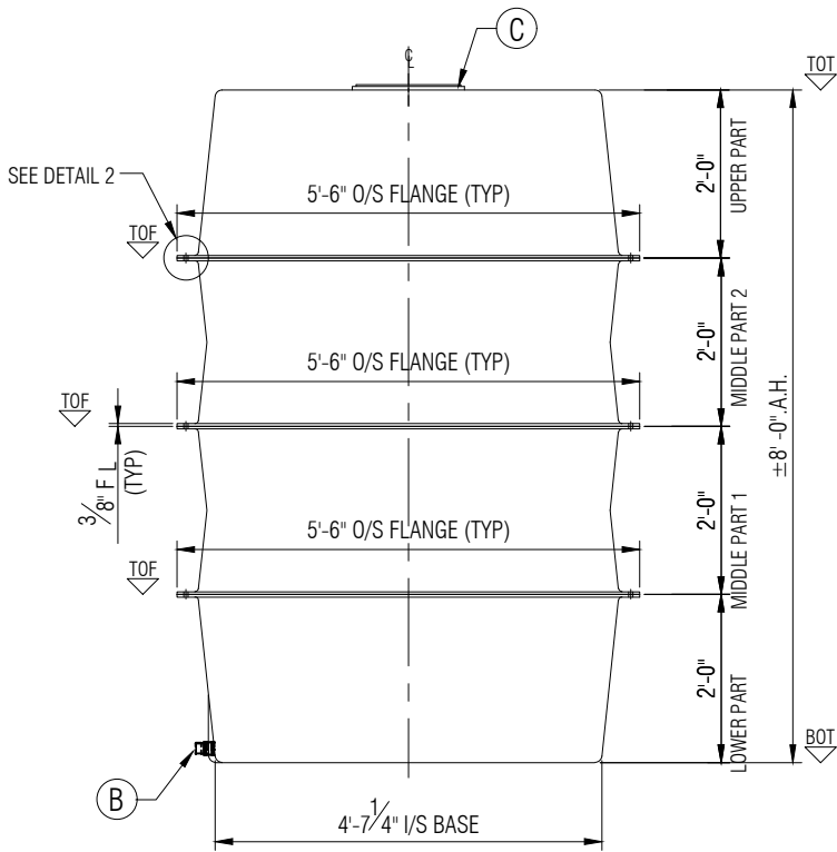
ELEVATION B
