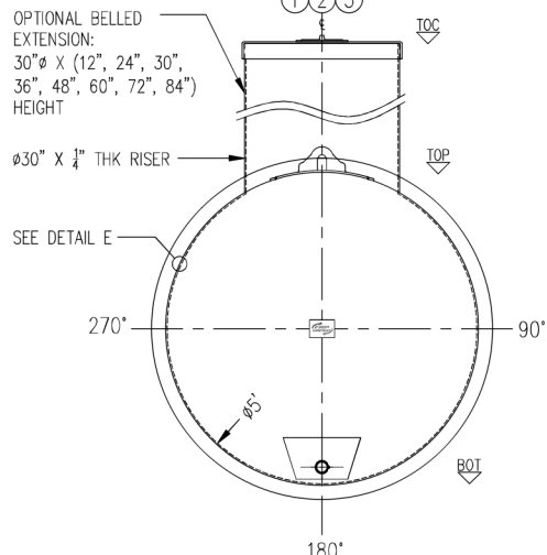
ELEVATION B
