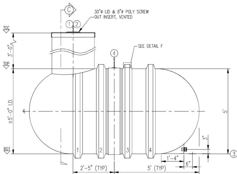
ELEVATION A
