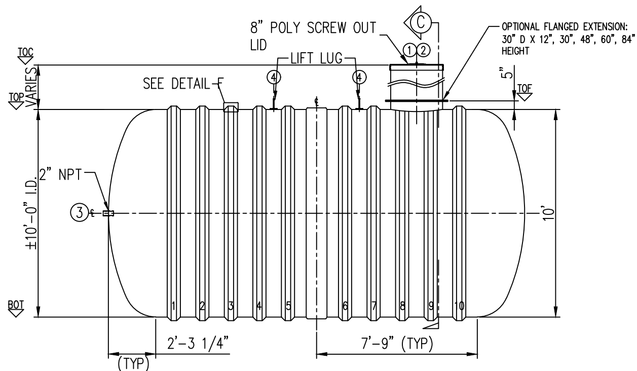
ELEVATION A
