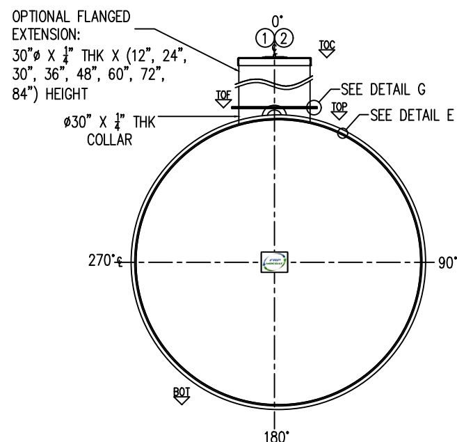
ELEVATION B
