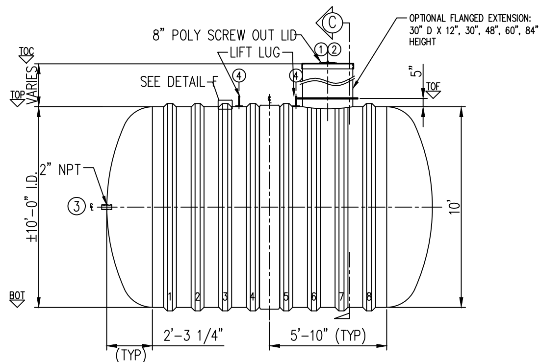
ELEVATION A
