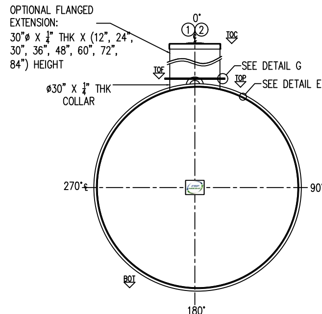
ELEVATION B
