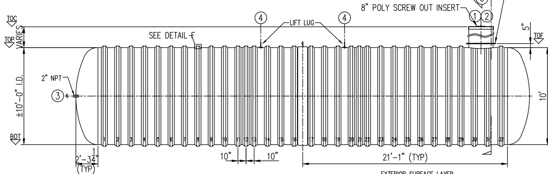
ELEVATION A
