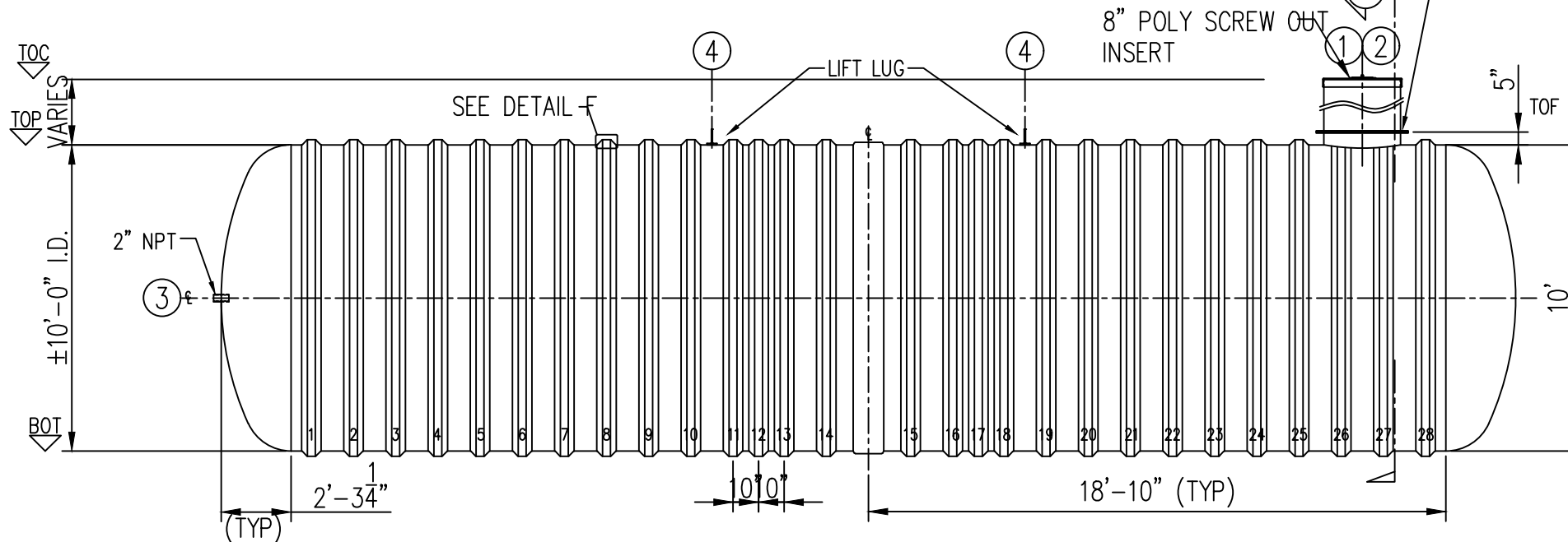
ELEVATION A
