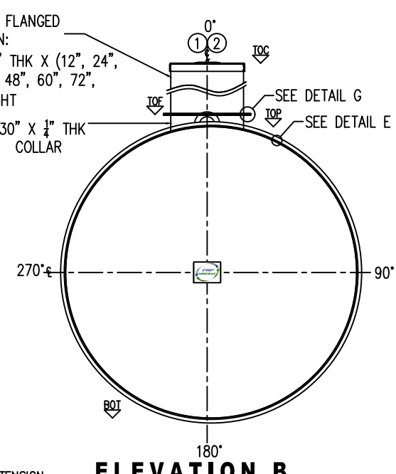
ELEVATION B
