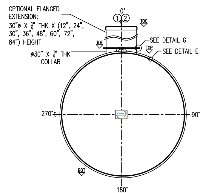
ELEVATION B
