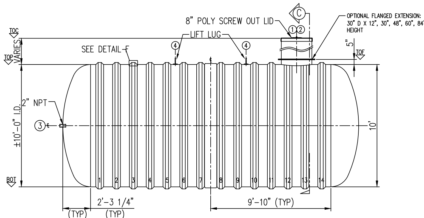
ELEVATION A
