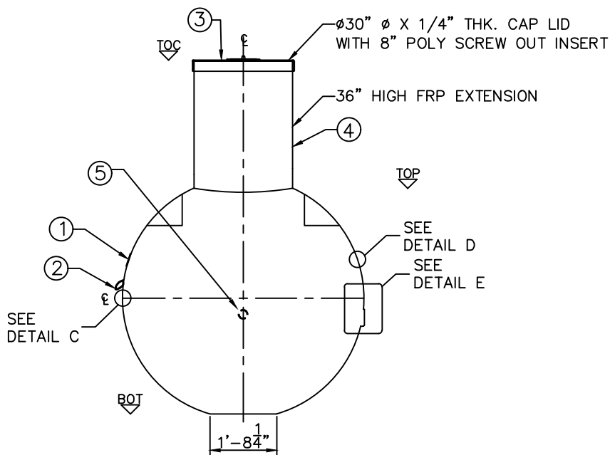
ELEVATION A
