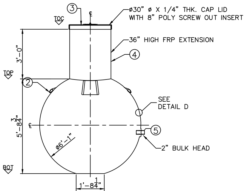
ELEVATION B
