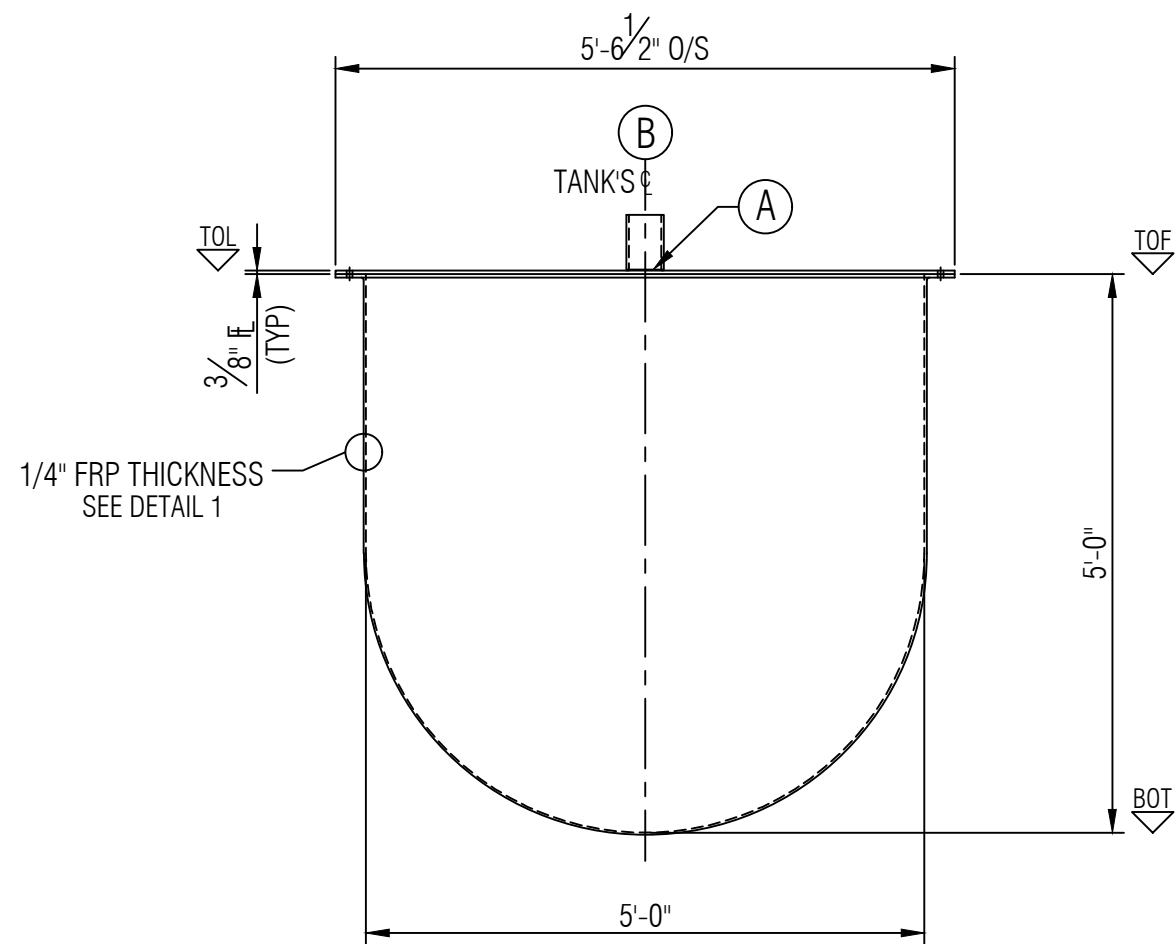
ELEVATION A
