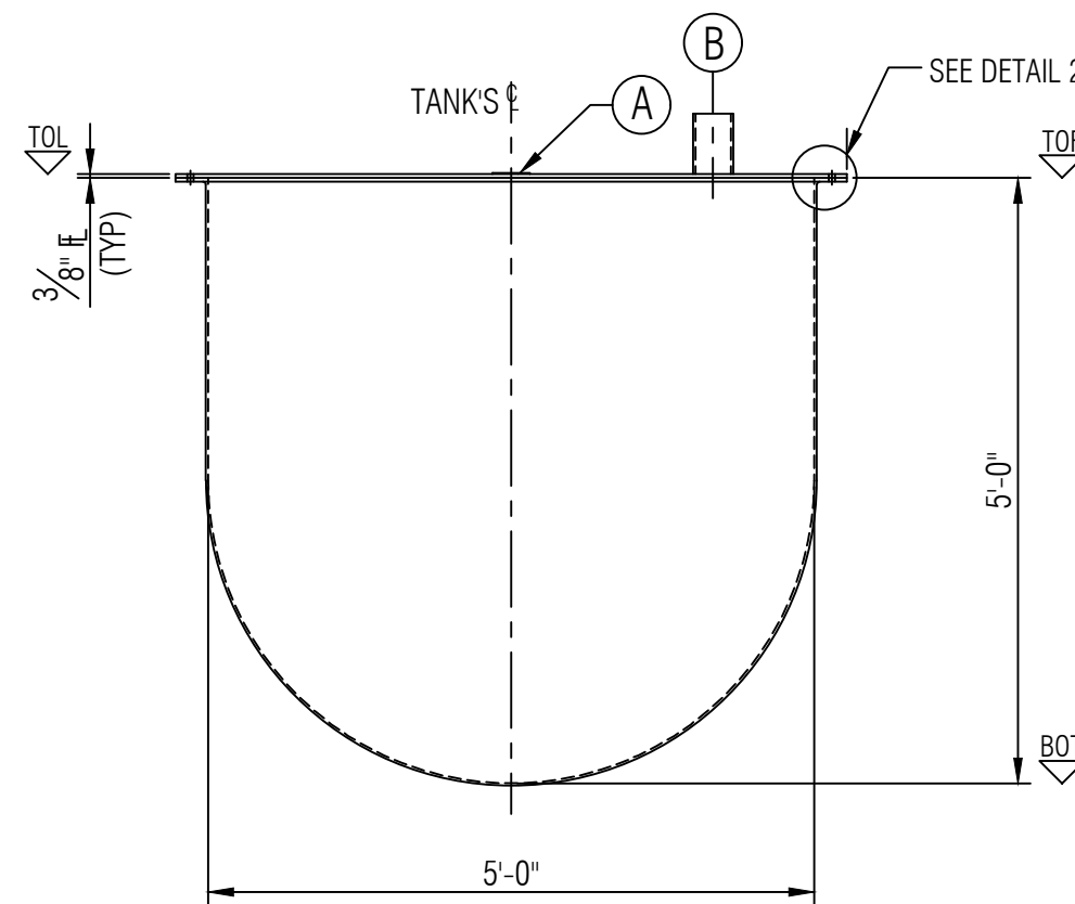
ELEVATION B
