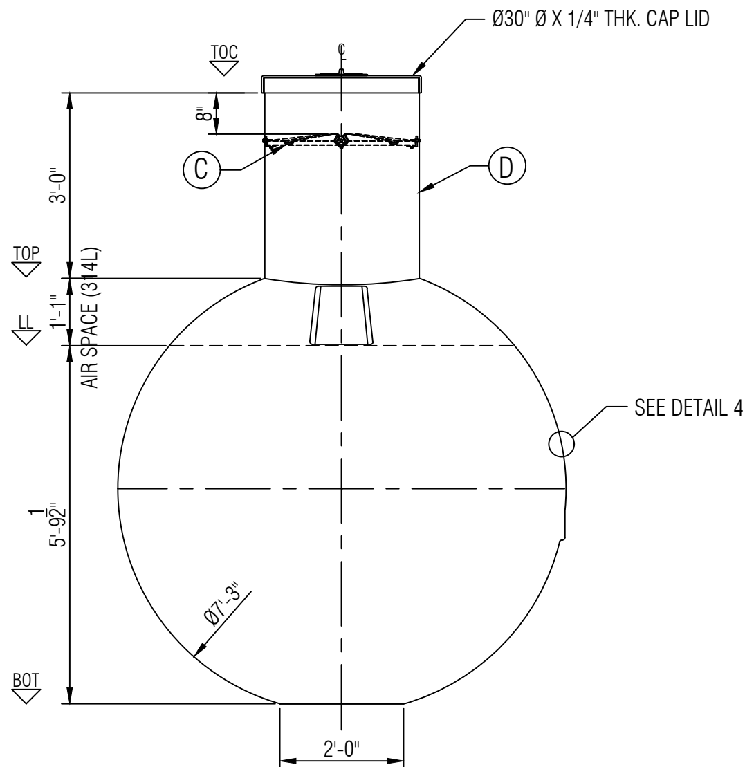
ELEVATION B
