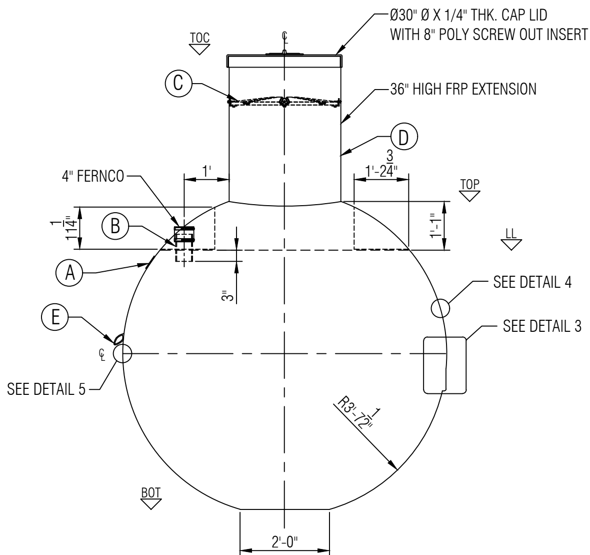
ELEVATION A
