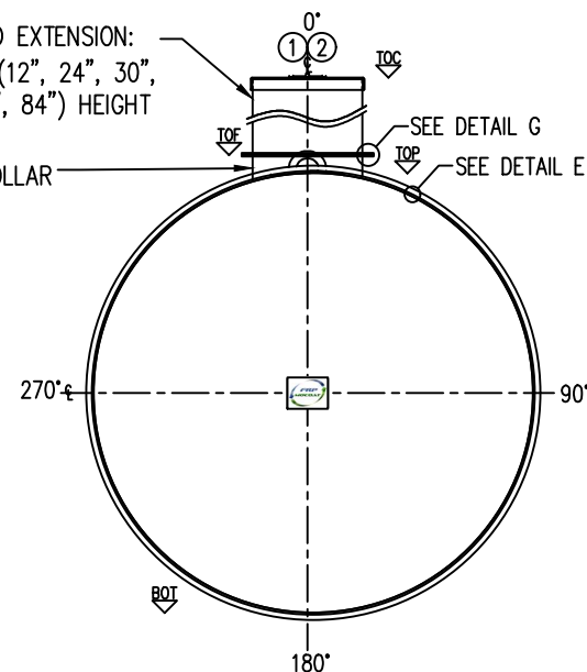
ELEVATION B
