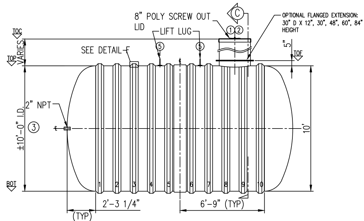
ELEVATION A
