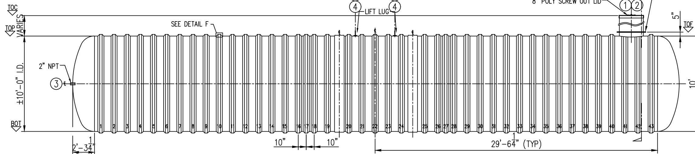
ELEVATION A
