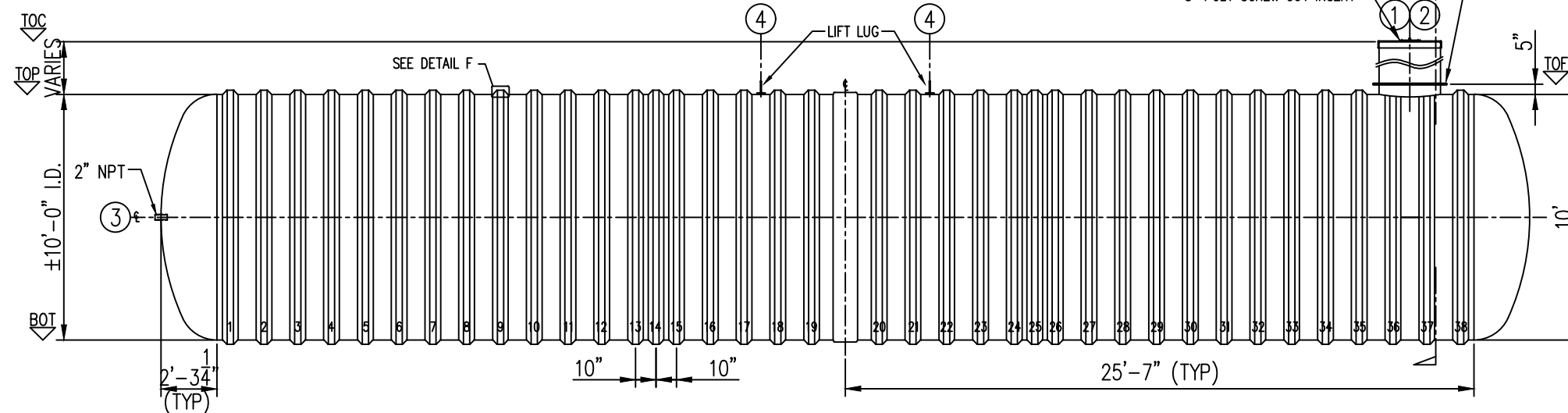
ELEVATION A
