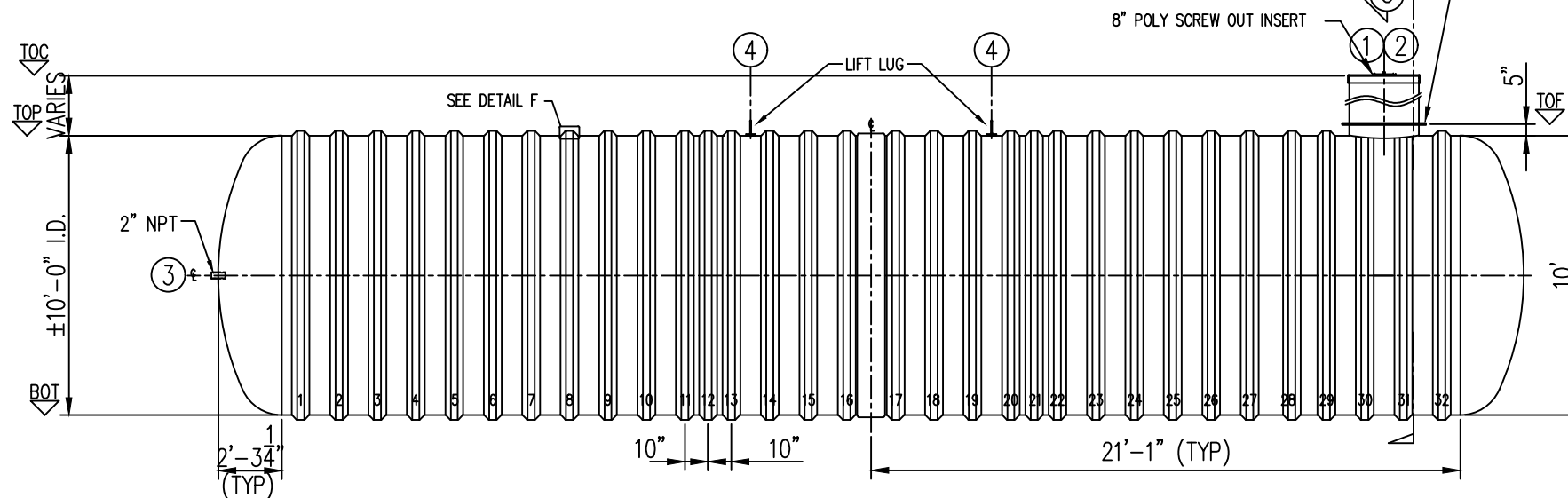
ELEVATION A
