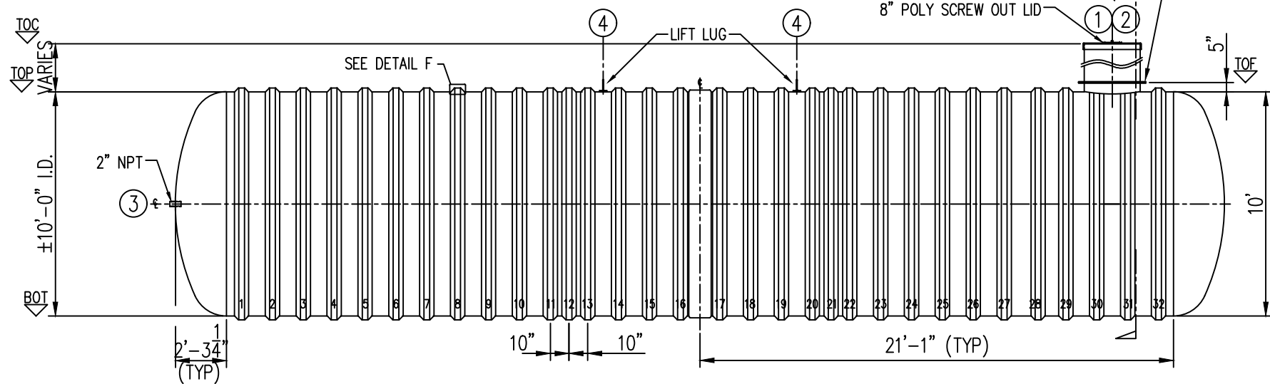
ELEVATION A
