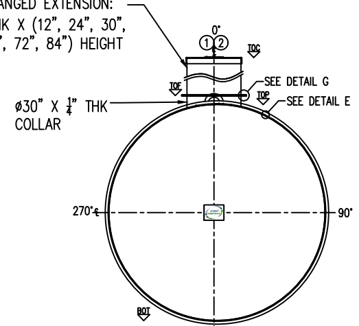
ELEVATION B
