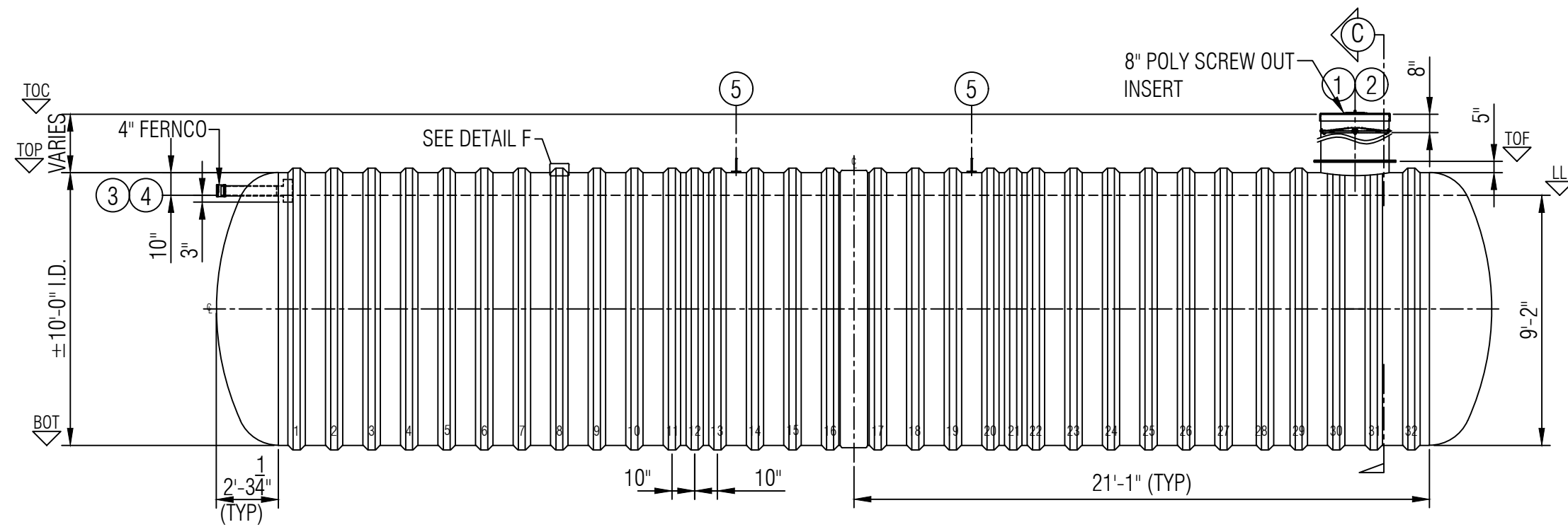
ELEVATION A
