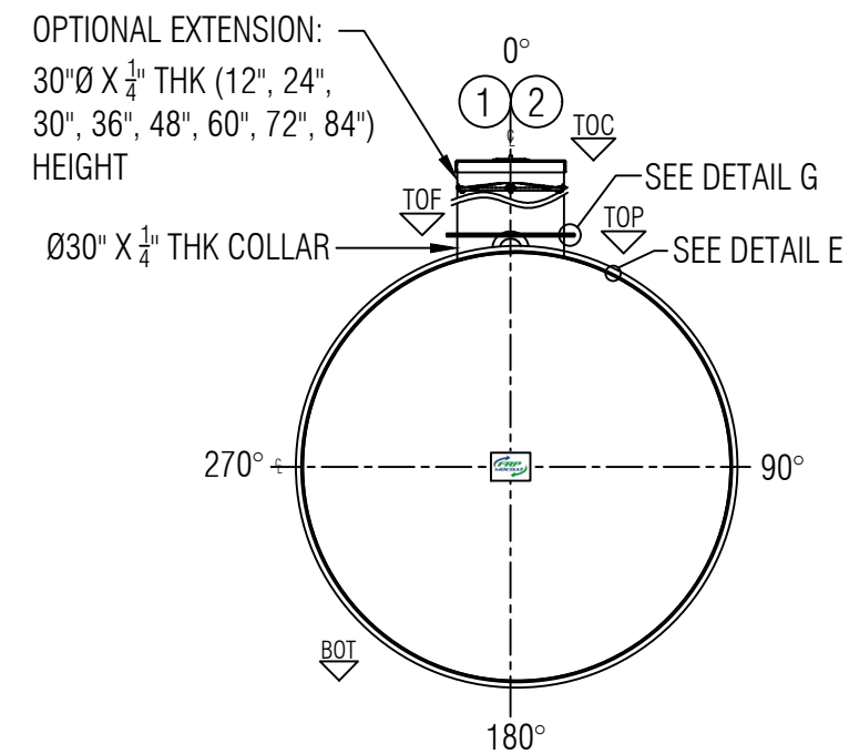
ELEVATION B
