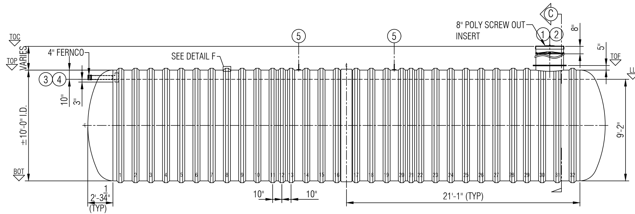
ELEVATION A
