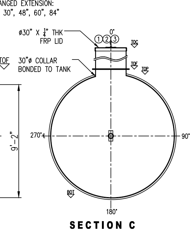
ELEVATION B
