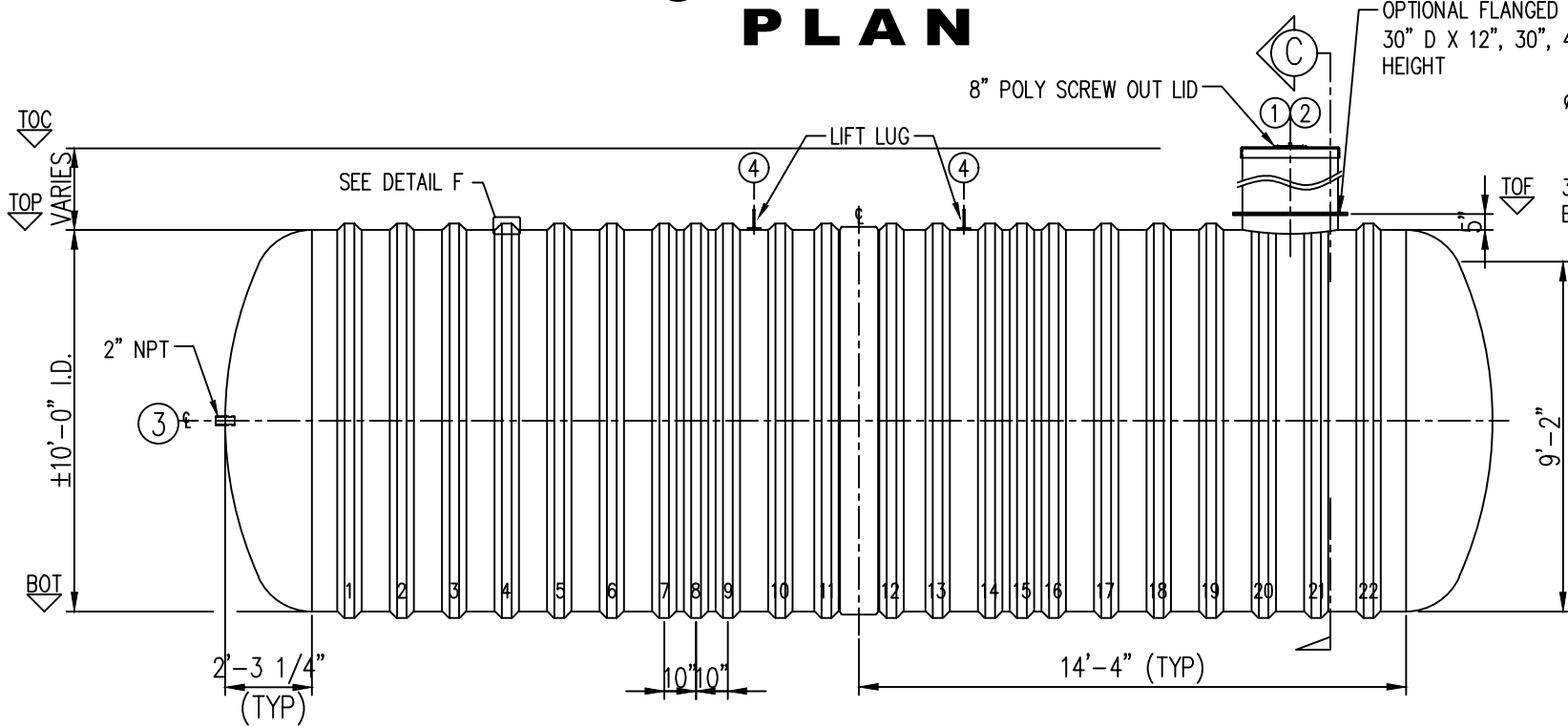
ELEVATION A
