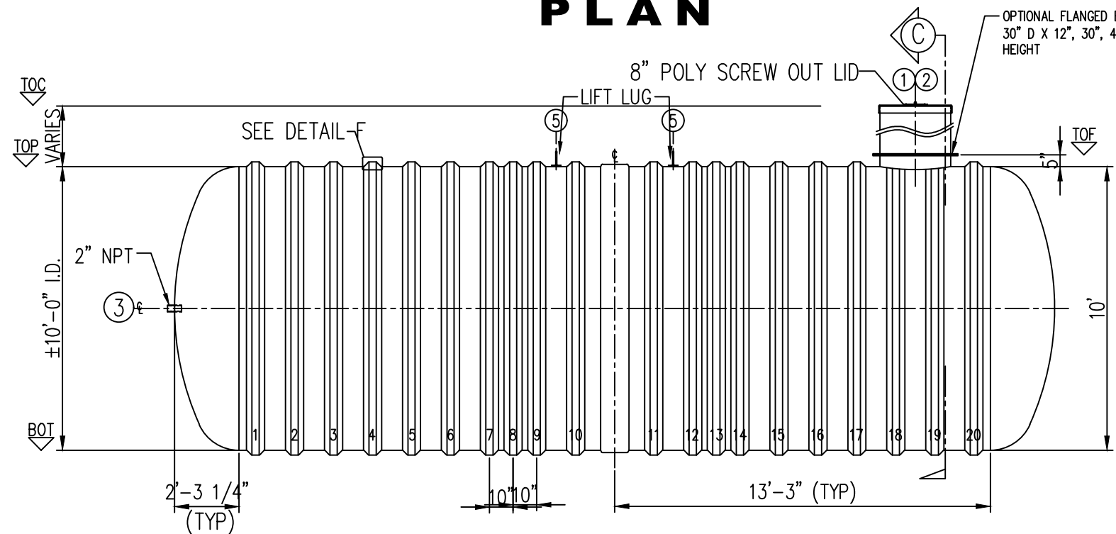
ELEVATION A
