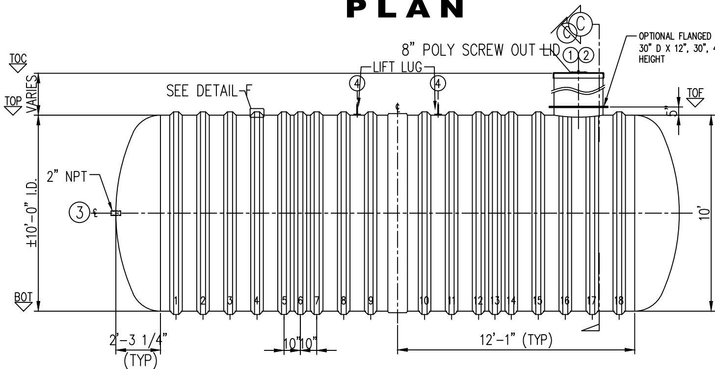
ELEVATION A
