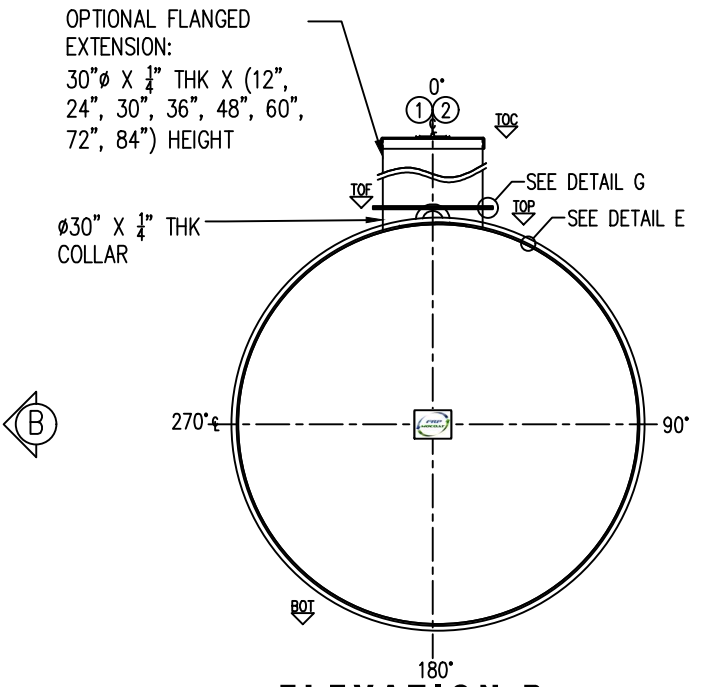
ELEVATION B
