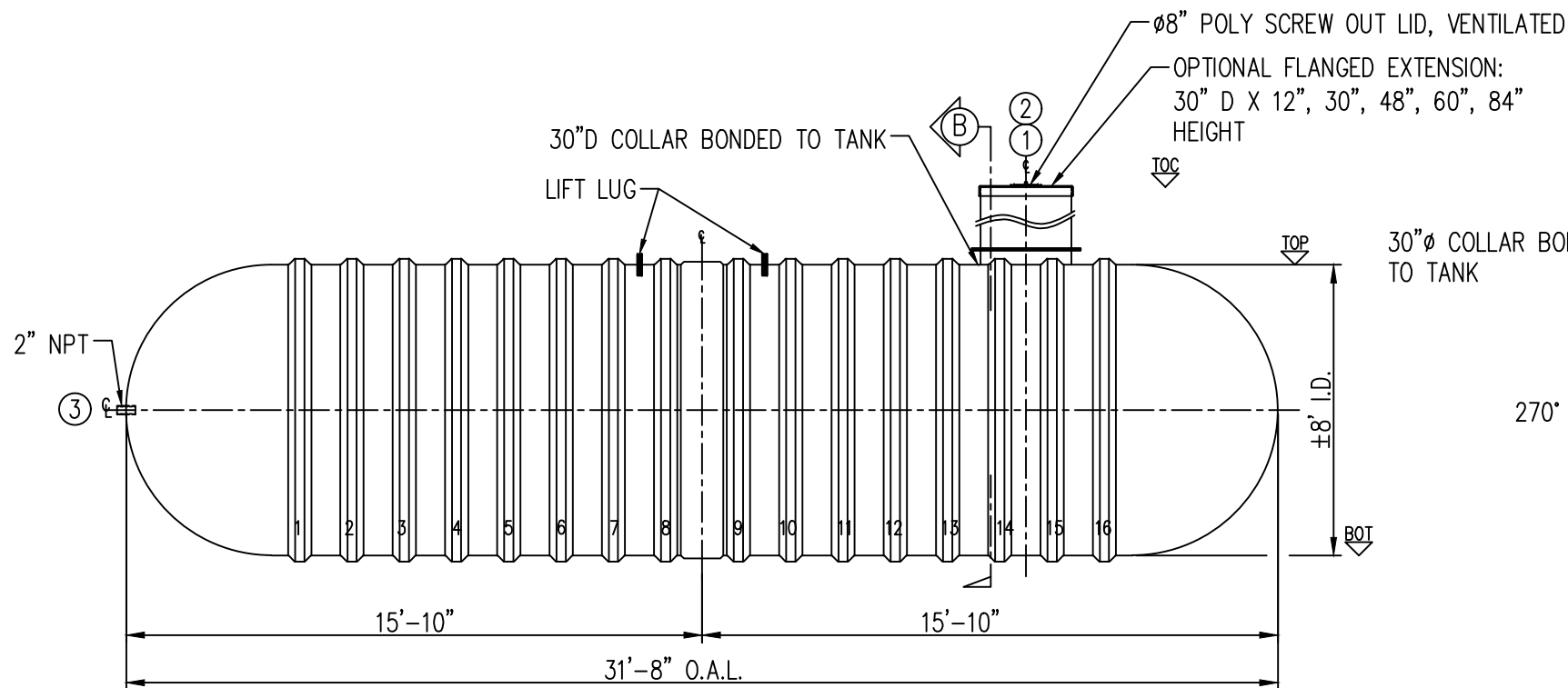
ELEVATION
