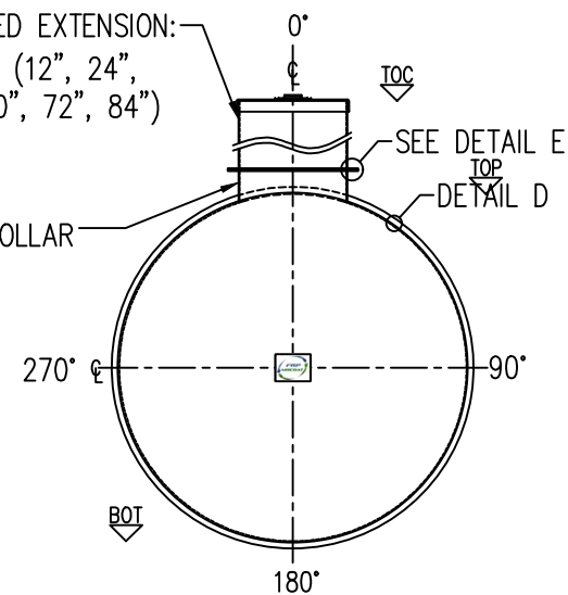
ELEVATION A
