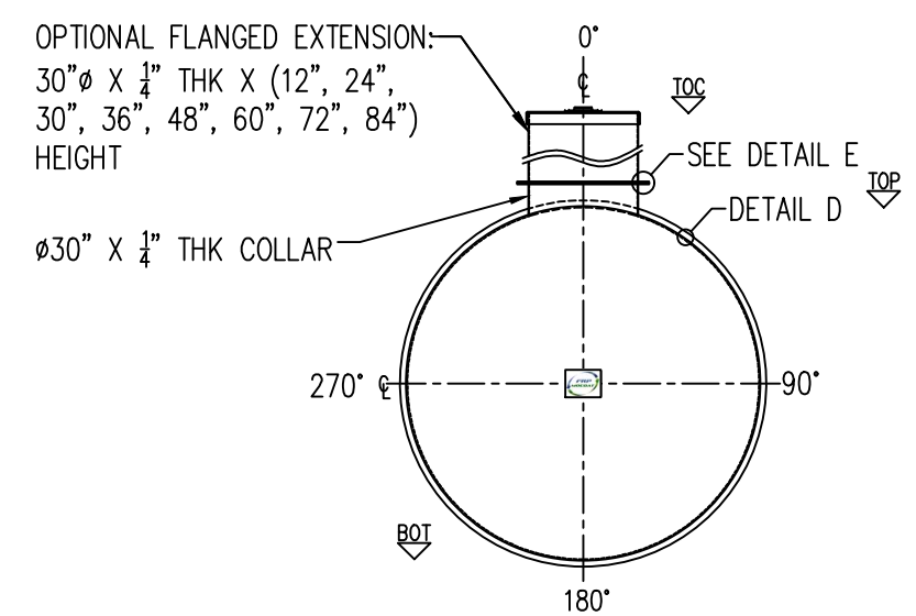
ELEVATION A
