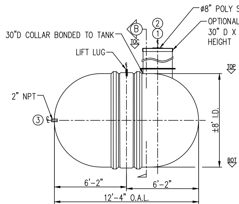
ELEVATION
