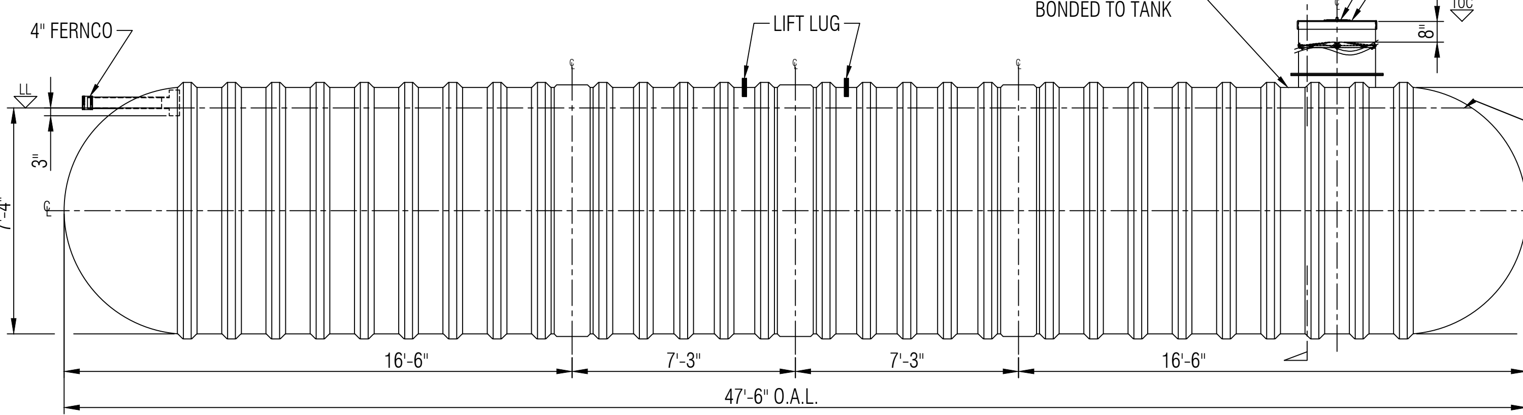
ELEVATION
