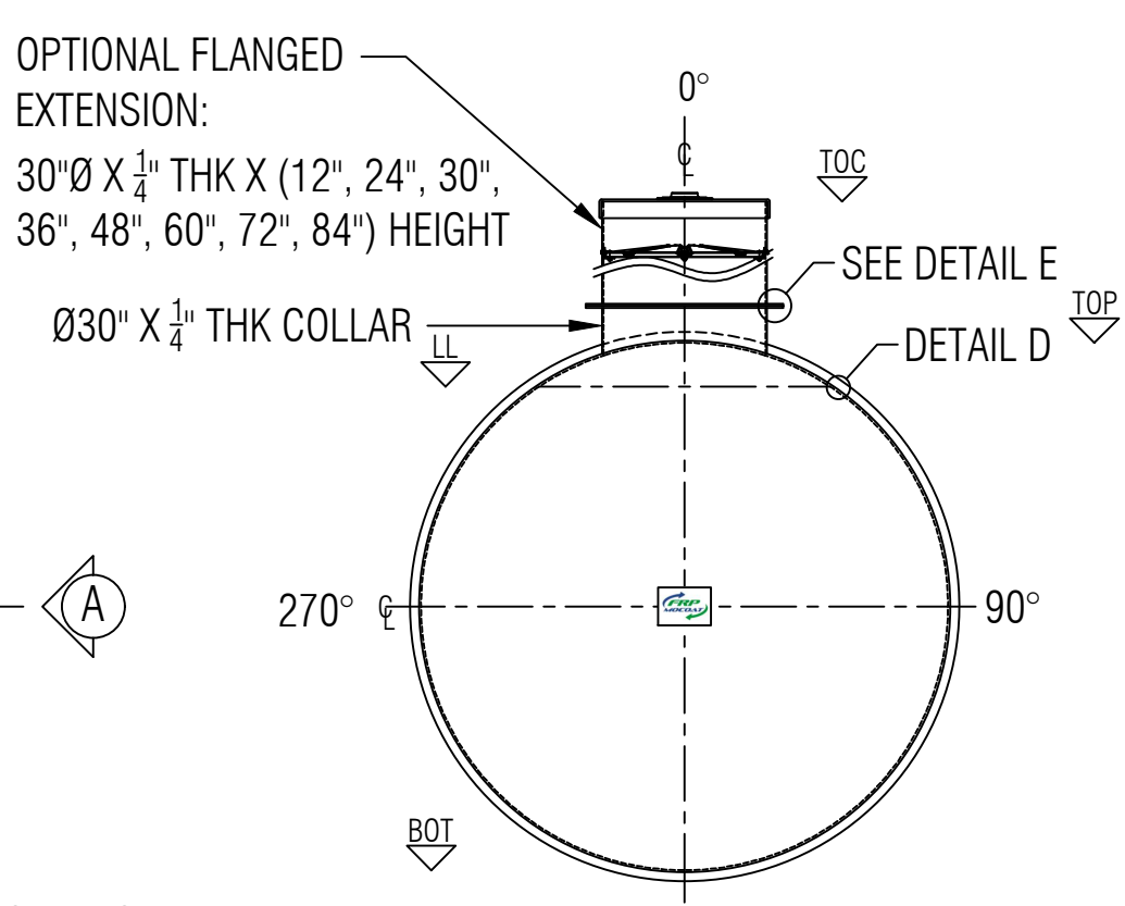
ELEVATION A
