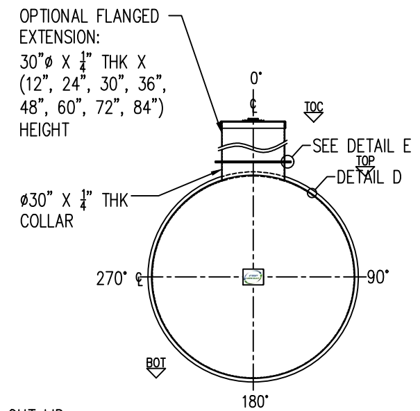
ELEVATION A
