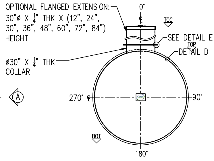
ELEVATION A
