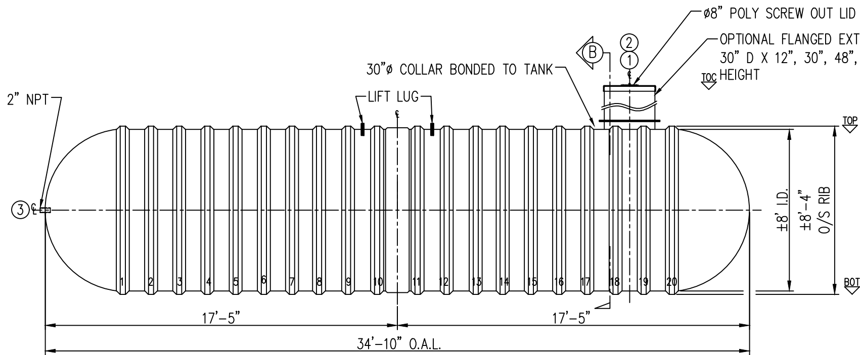
ELEVATION
