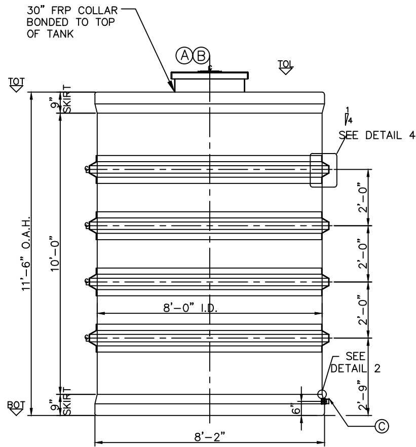
ELEVATION B
