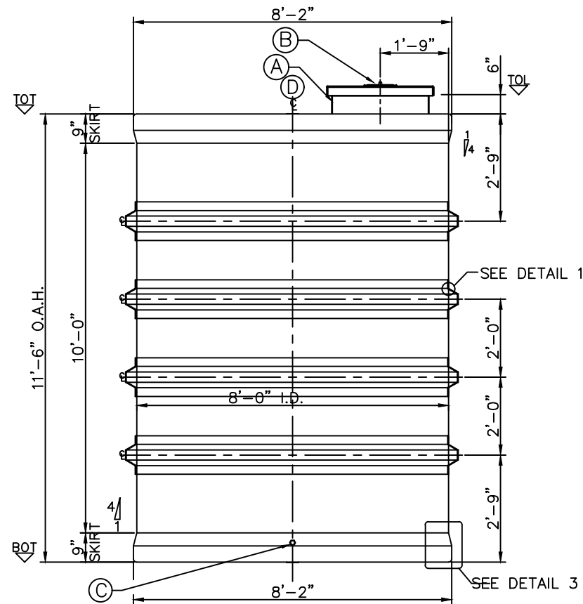
ELEVATION A
