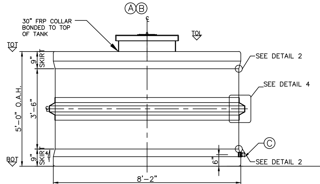
ELEVATION B
