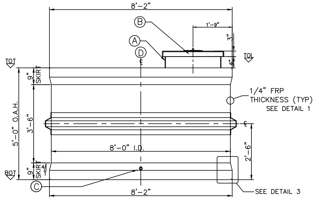
ELEVATION A
