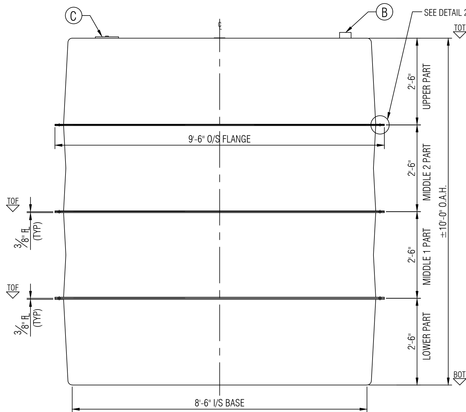
ELEVATION B
