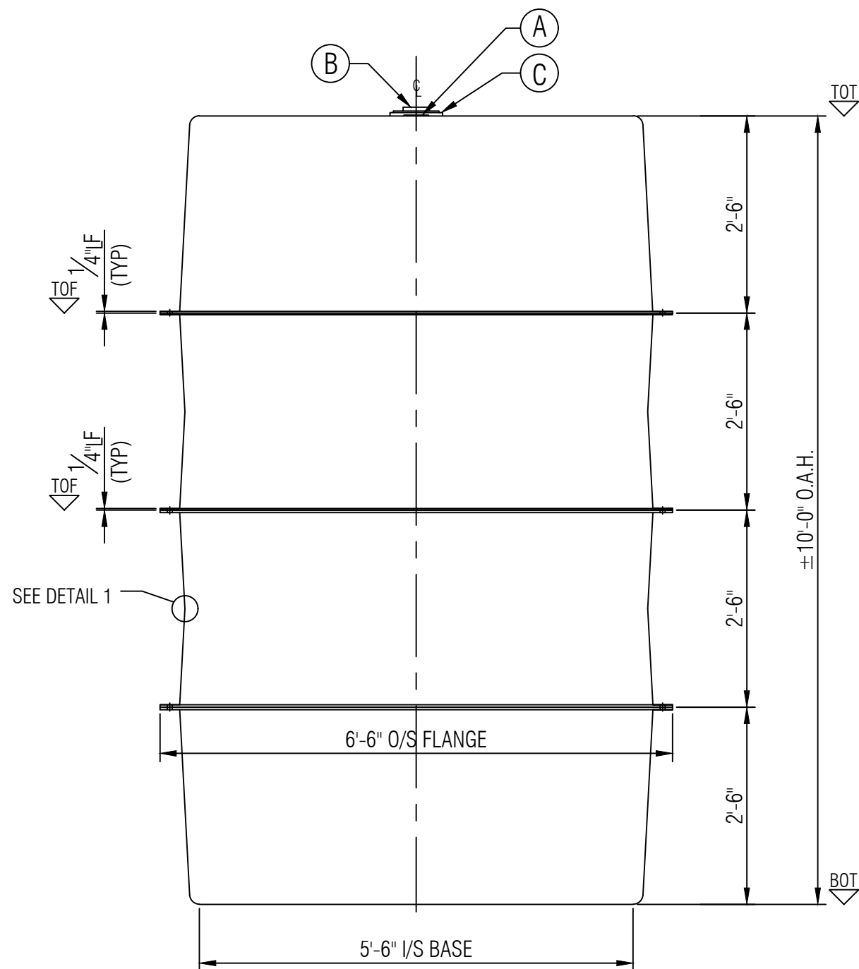
ELEVATION A
