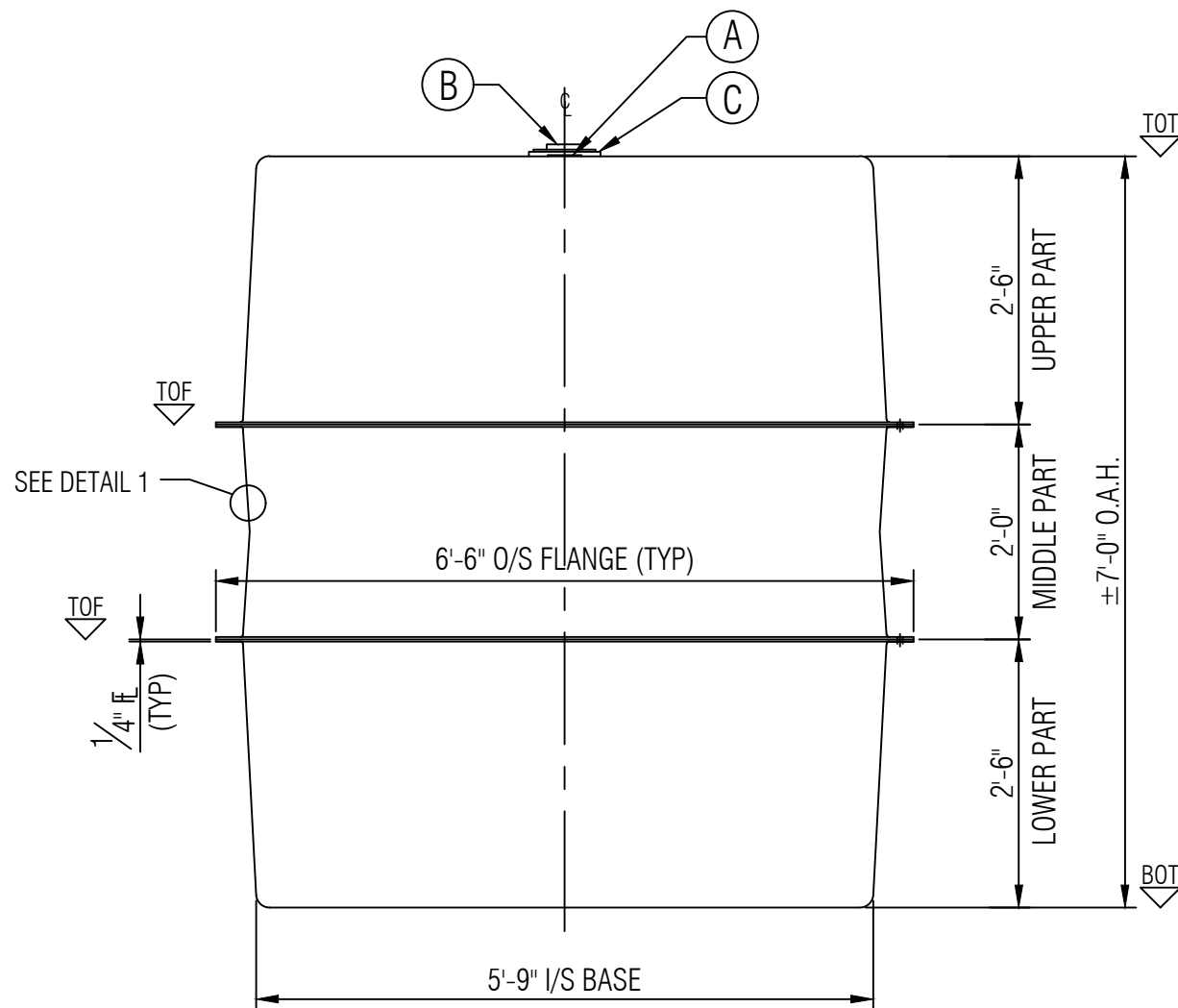
ELEVATION A
