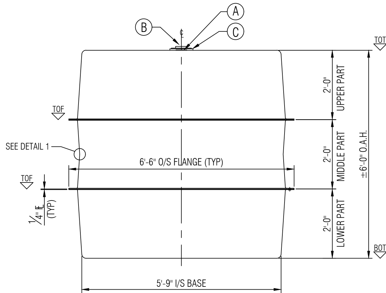
ELEVATION A
