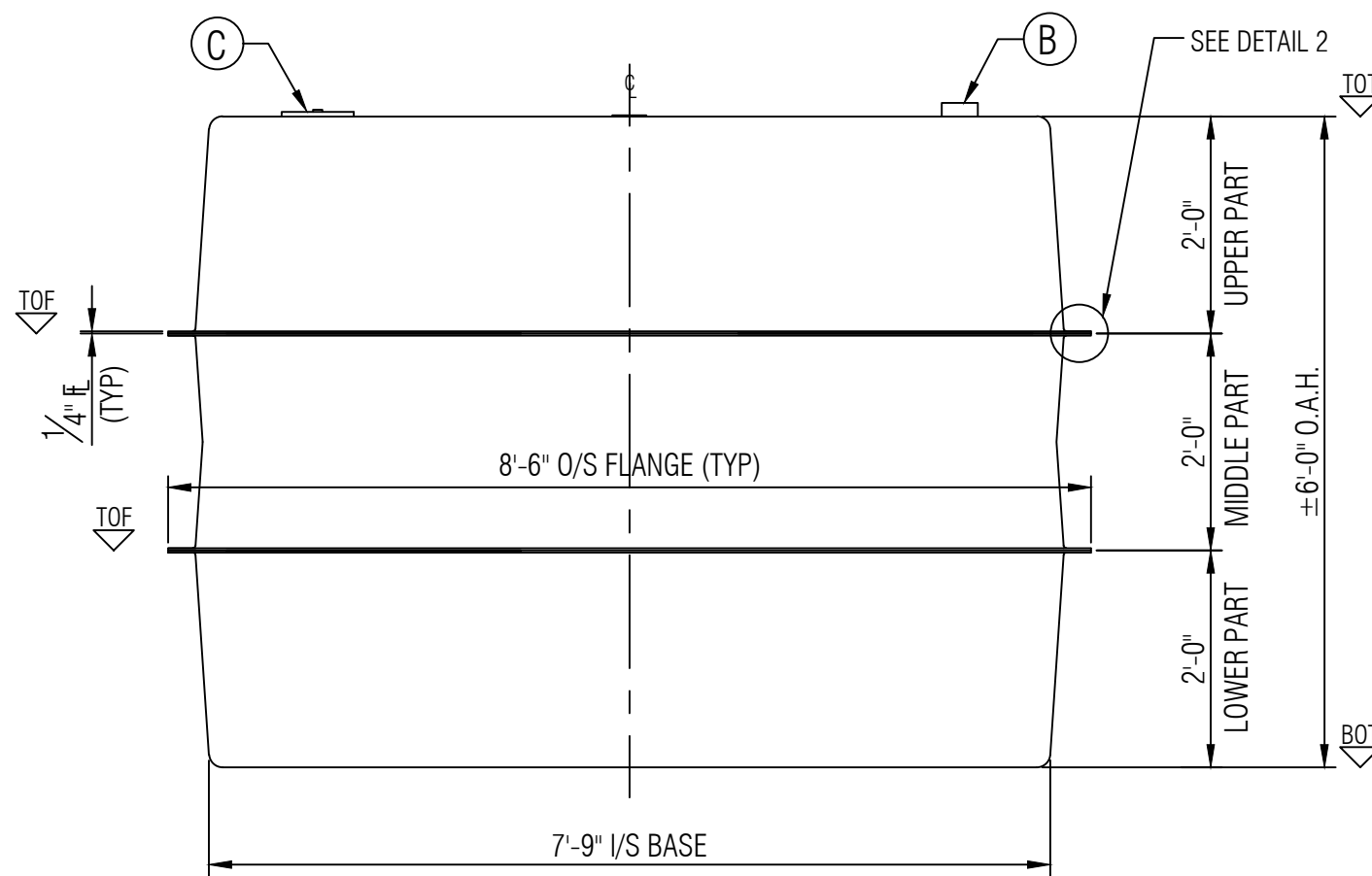
ELEVATION B
